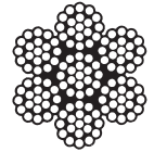
6 x 19 (1+6+12) + SEL
