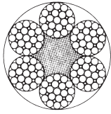
6 x 19 Filler + FE
