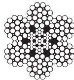
6 x 19 Filler + SES
