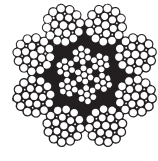
8 x 19 Filler (1+6+6F+12) + SES
