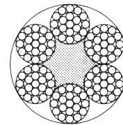
6 x 19 (1+6+12) + FE
