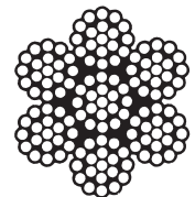
6 x 19 (1+6+12) + SEL
